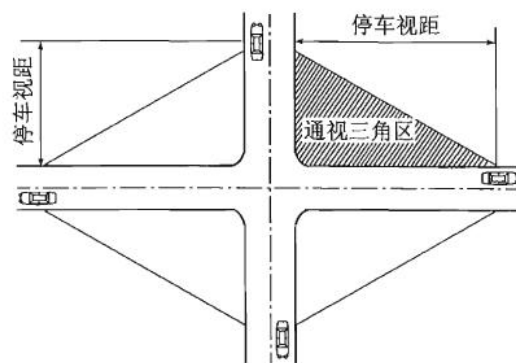
图 10.0.8-2 通视三角区
