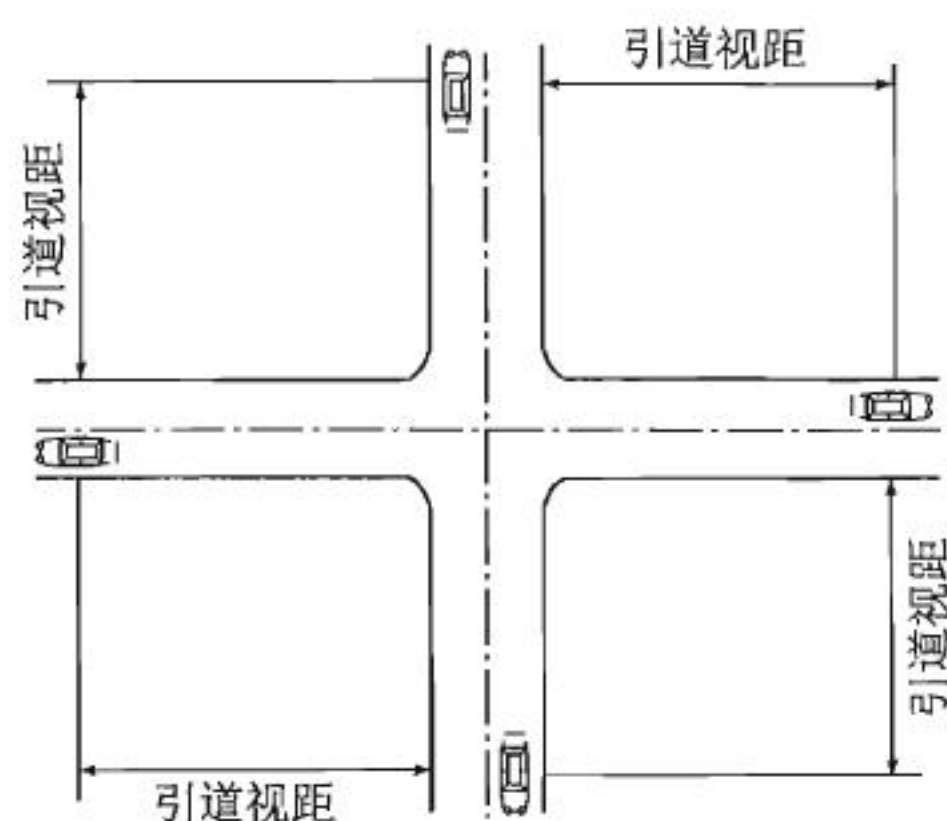
图 10.0.8-1 引道视距
