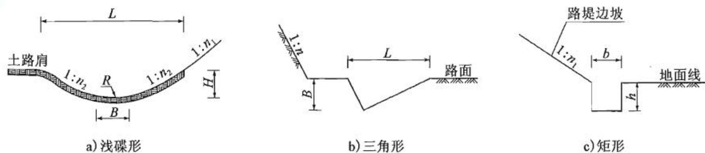
图 7.0.2 典型边沟或排水沟形式
