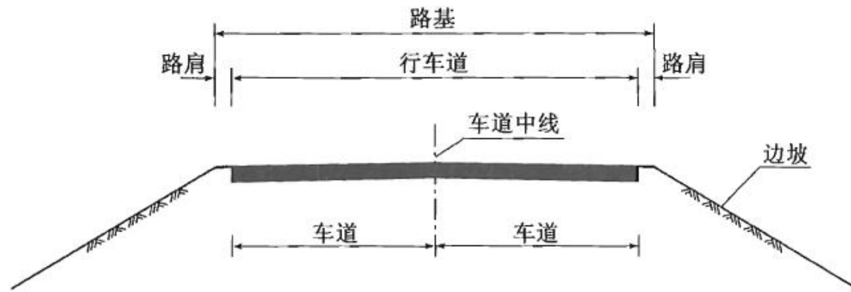
图 4.0.4-1 四级公路 (I类) 典型横断面
