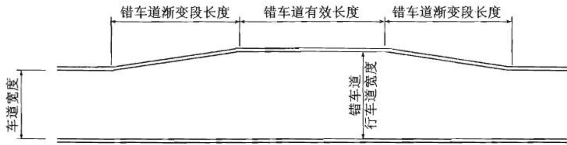
图 4.0.3 错车道平面布置图
