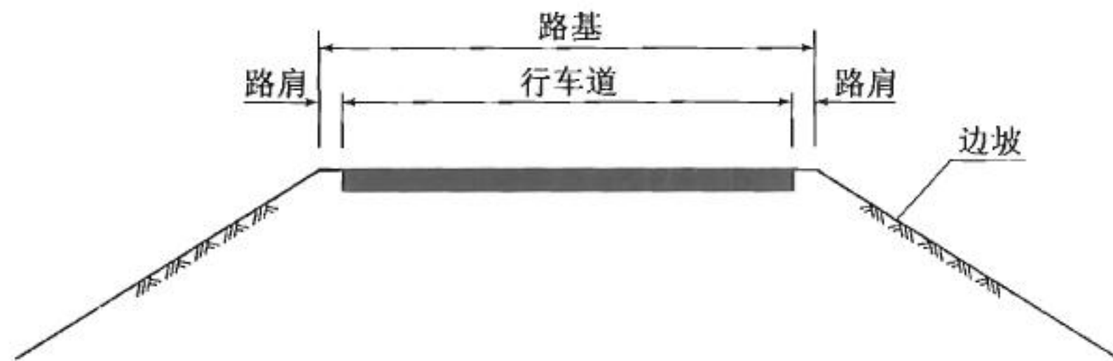
图 4.0.4-2 四级公路 (II类) 典型横断面
