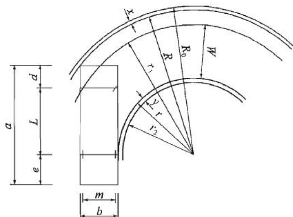
图 4-1 圆曲线最小半径计算示意图
