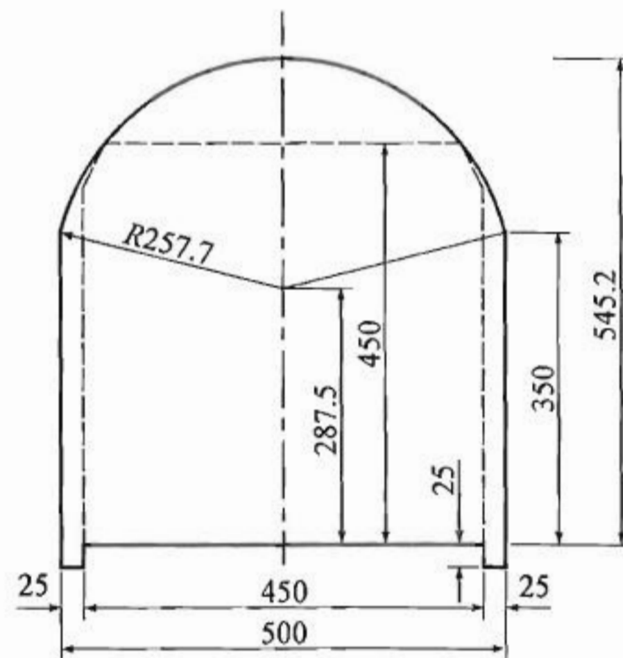
图 B.0.2 单车道隧道直墙式衬砌标准内轮廓断面 (尺寸单位: cm)
