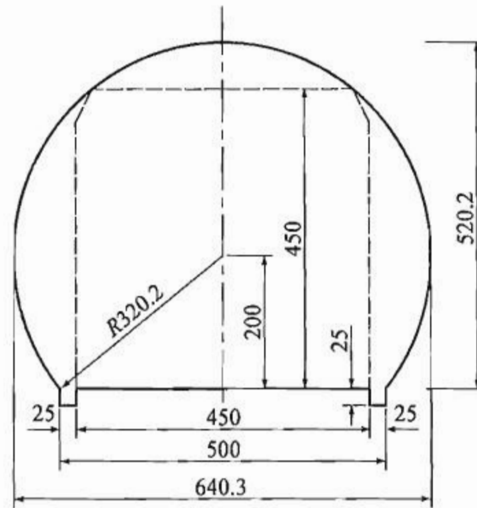
图 B.0.1 单车道隧道曲墙式衬砌标准内轮廓断面 (尺寸单位: cm)
