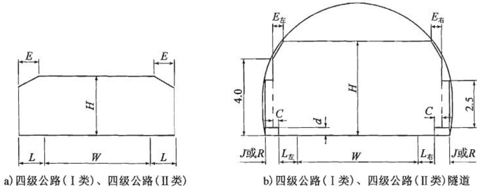
图 3.5.1 四级公路（I类）、四级公路（II类）建筑限界（尺寸单位：m）
