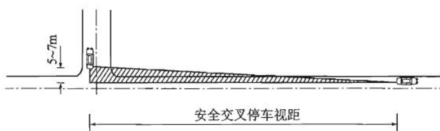
图 10.0.8-3 安全交叉停车视距通视三角区
